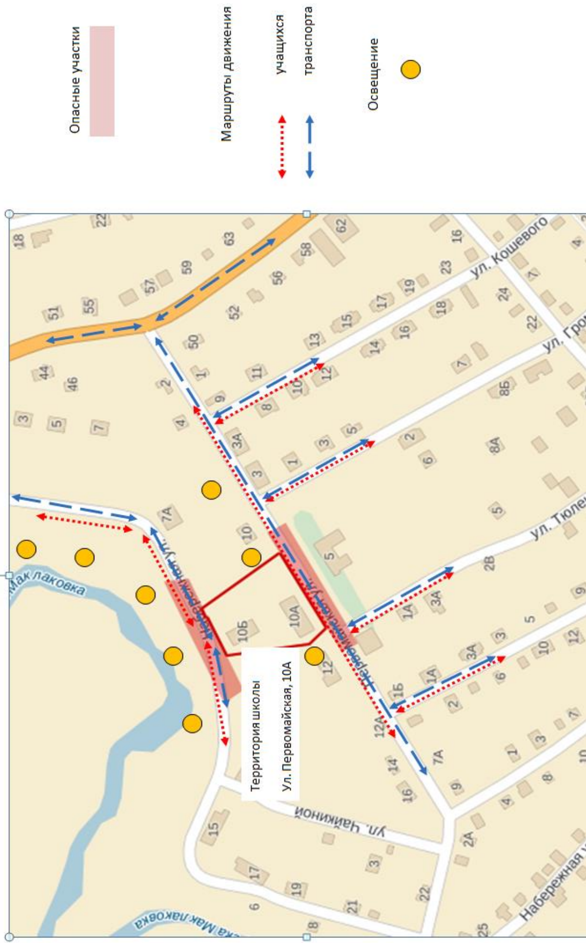
Схема организации дорожного движения в непосредственной близости от образовательного учреждения (ул. Первомайская, 10А)
